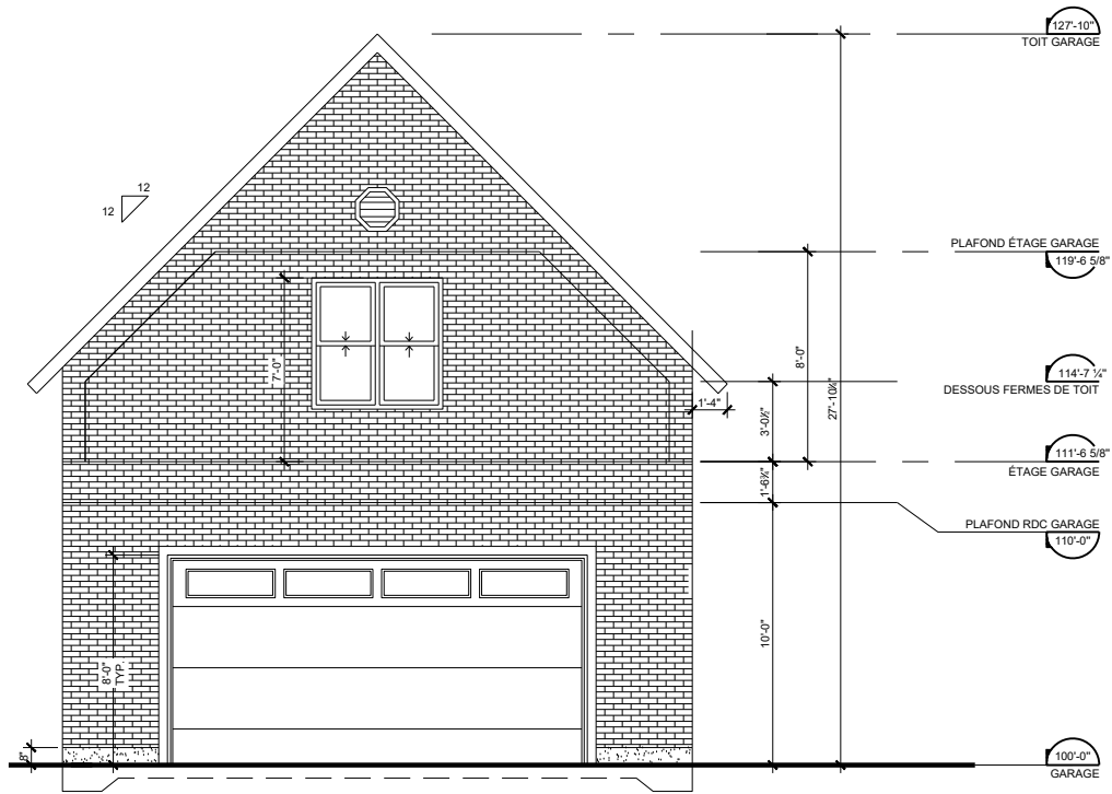
1 ÉLEVATION AVANT 1/4"=1'-0"
