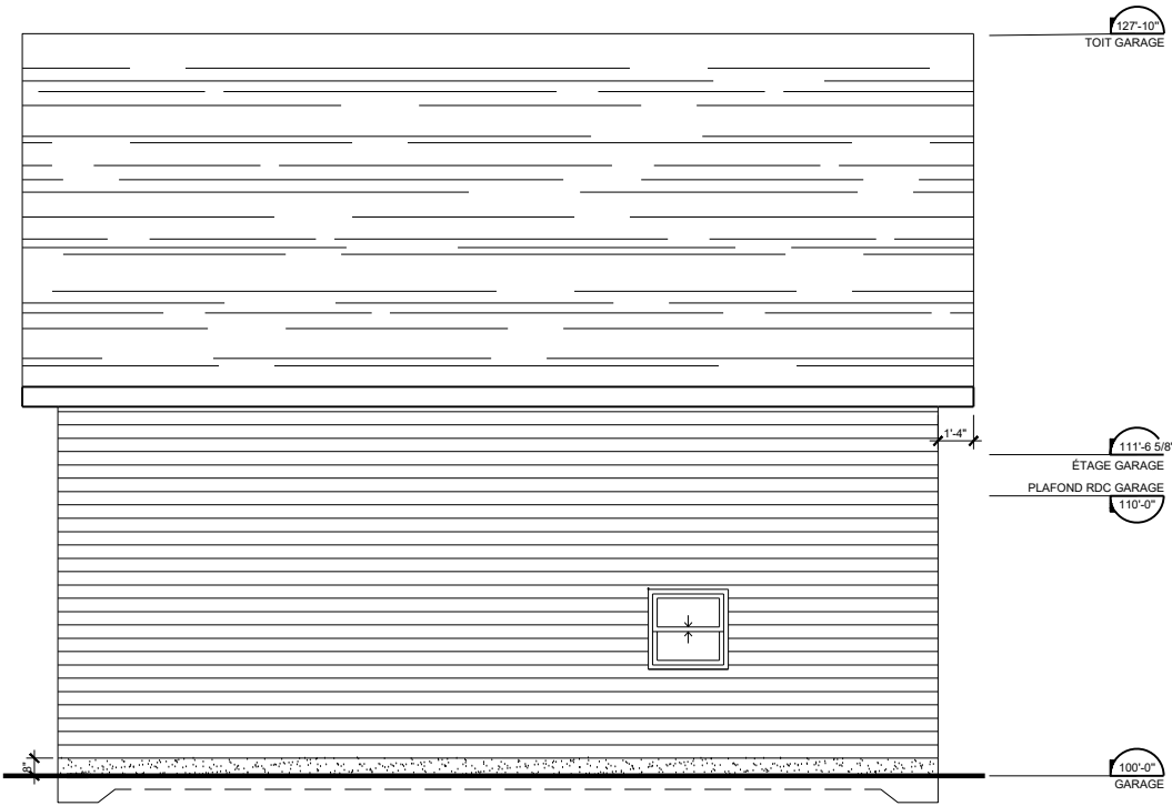
4 ÉLEVATION DROITE 1/4"=1'-0"
