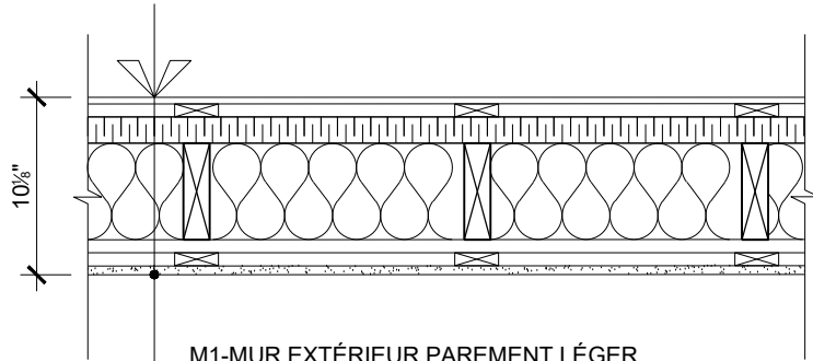
M1-MUR EXTÉRIEUR PAREMENT LÉGER
