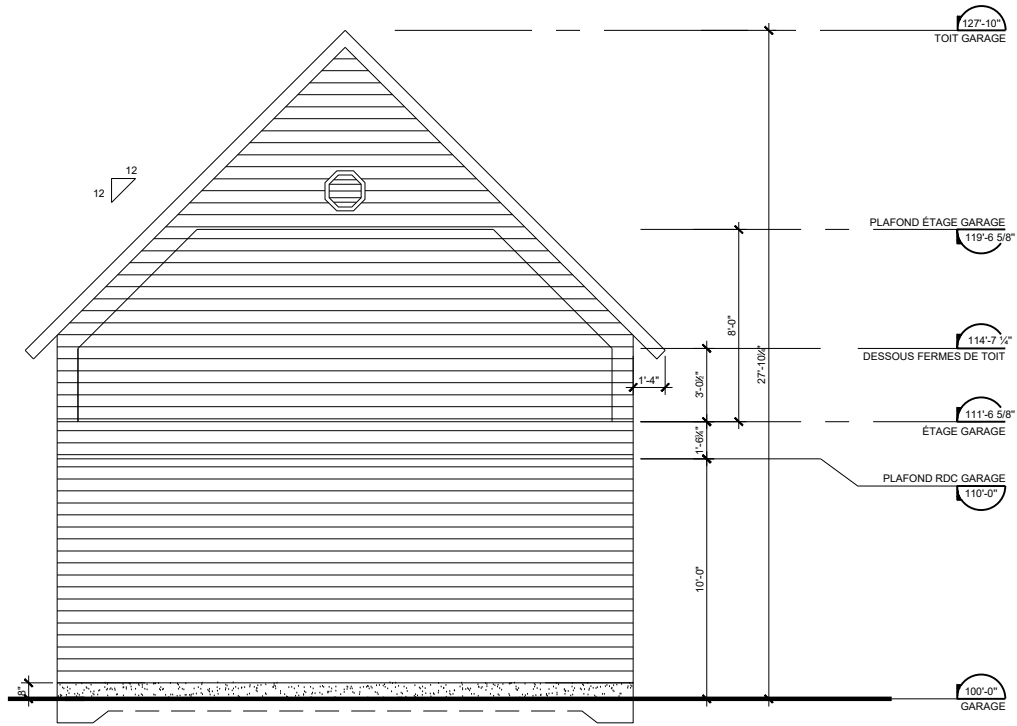
2 ÉLEVATION ARRIÈRE 1/4"=1'-0"
