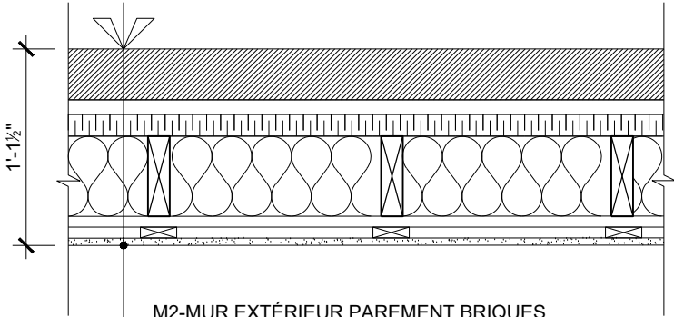
M2-MUR EXTÉRIEUR PAREMENT BRIQUES
