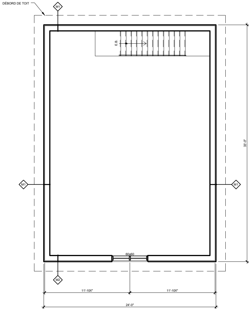
2 PLAN ÉTAGE 10 1/4"=1'-0"
