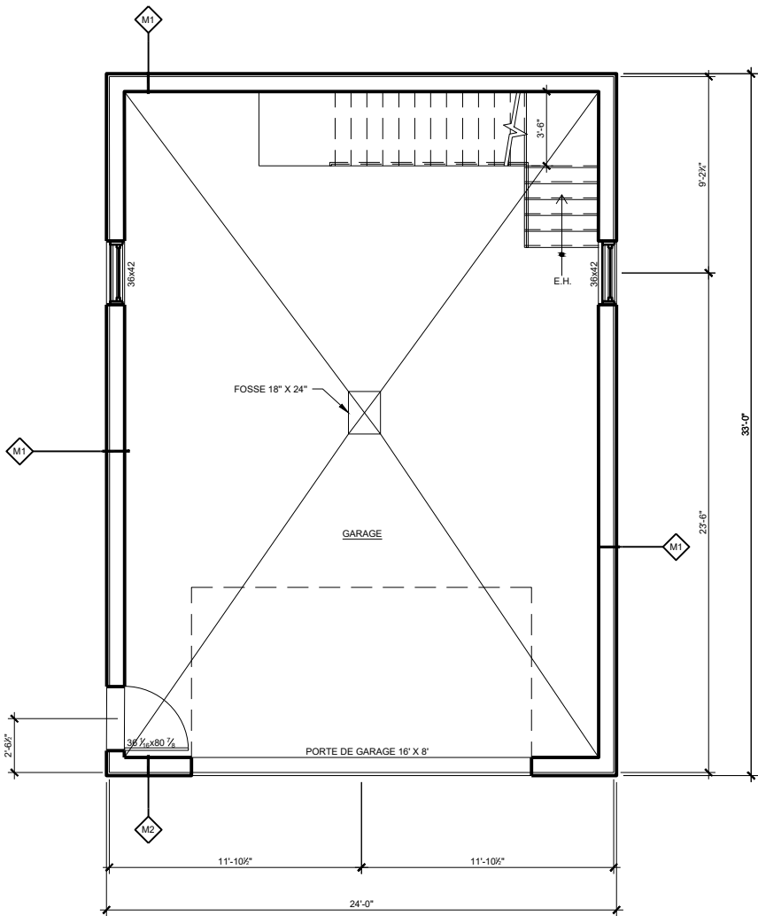
1 PLAN RDC 10 1/4"=1'-0"
