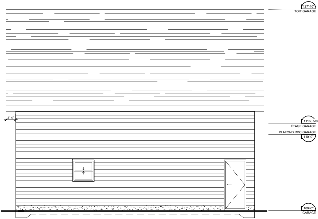
3 ÉLEVATION GAUCHE 1/4"=1'-0"
